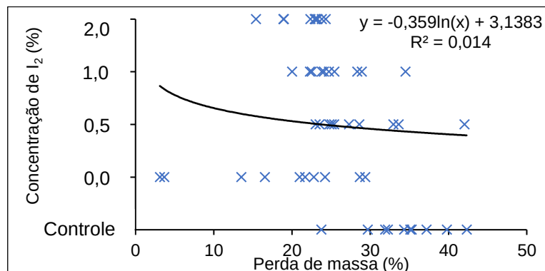
Figura 2. Perda de massa (%) causada pelo fungo Gloeophyllum trabeum para as concentrações de iodo no óleo de soja.
