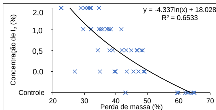
Figura 1. Perda de massa (%) causada pelo fungo Rhodonia placenta para as concentrações de iodo no óleo de soja.
