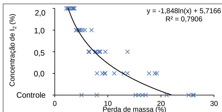
Figura 3. Perda de massa (%) causada pelo fungo Trametes versicolor para as concentrações de iodo no óleo de soja.
